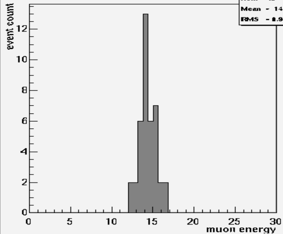
Muon Energy
